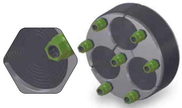
Stufenlose Scheibentechnik! Beispiel KRASO® Dichteinsatz Universal Mehrfach 150 - geteilt - Ausführung 1: 3 x 6 - 52 mm oder blind
